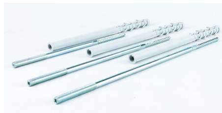
Kombiskrutky s hmoždinkou v rôznych veľkostiach: 8 x 80, 8 x 140, 8 x 200, 8 x 250 a 8 x 300
